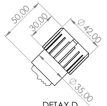
DETAY D ÖLÇEK 1 : 2
