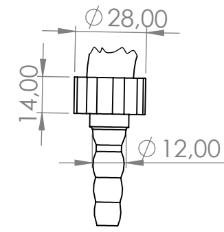
DETAY B ÖLÇEK 1 : 2
