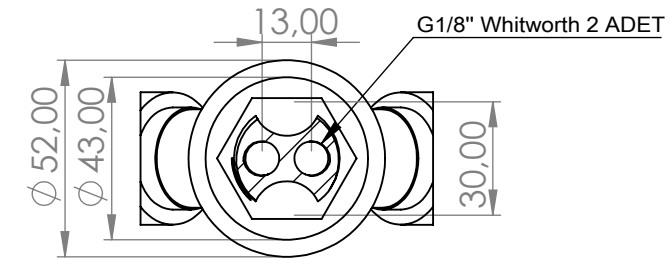
KESİT F-F ÖLÇEK 1 : 2
