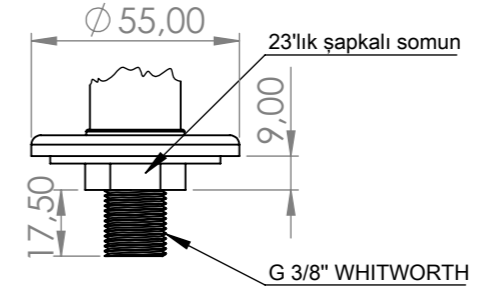
DETAY E ÖLÇEK 1 : 2
