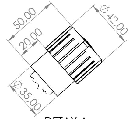
DETAY A ÖLÇEK 1 : 2
