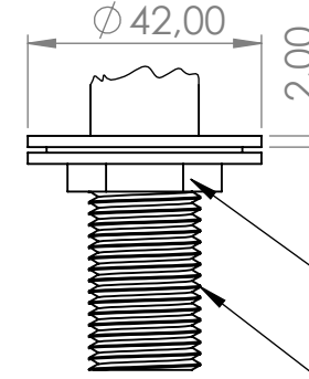
DETAY C ÖLÇEK 2 : 3
