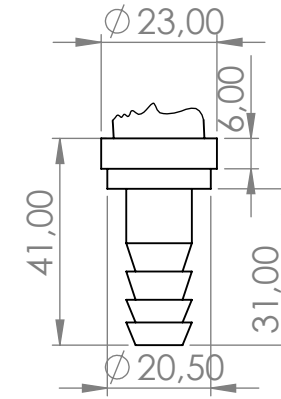
DETAY A ÖLÇEK 2 : 3
